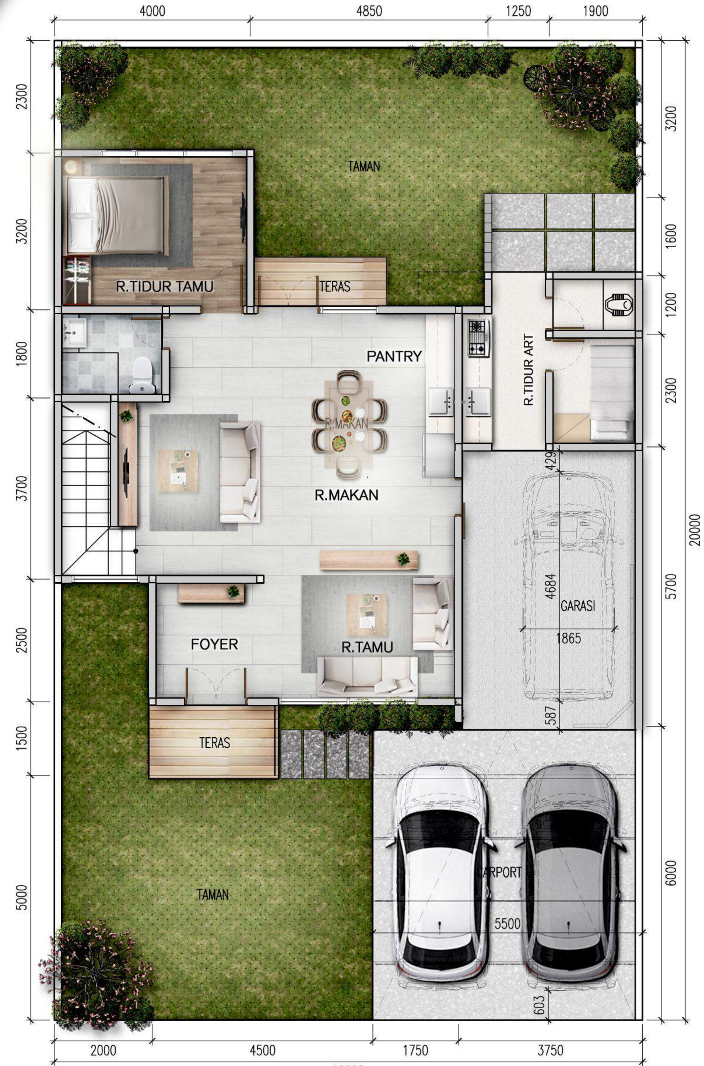
1 DENAH LT. SATU SKALA 1:100 (114m 2 ) HOOK
